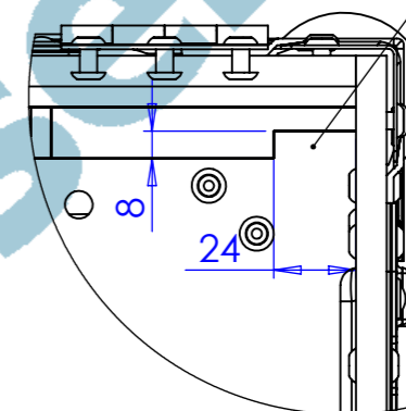
DETAIL F MĚŘITKO 5 : 12
